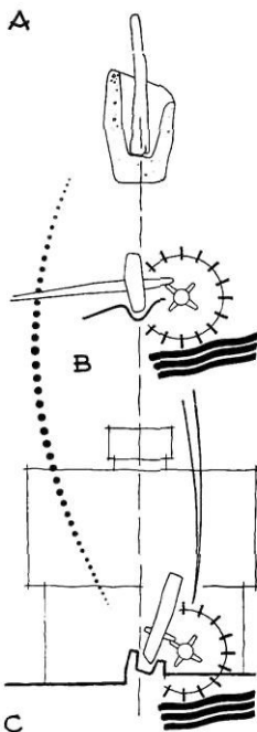
3. ábra A víz mozgásenergiájának felhasználása útő rendszerű — szakaszos munka-mozgású — munkaeszköz működtetésére. A mozsár, B függőleges forgássíki vizikerek, C kalapács (kölyű) malom
