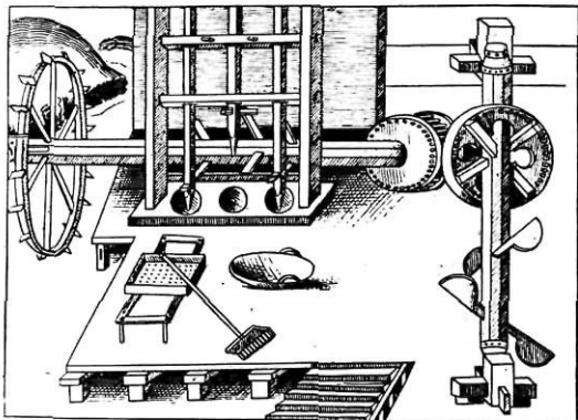
124. ábra Olajütőmalom vázlata a XV. sz.-ból (Walzburg – Wolfegg Hausbuch, 1480 körül)
