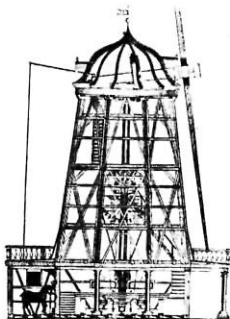
153. ábra. Galériás-tornyos szélmalom metszete
