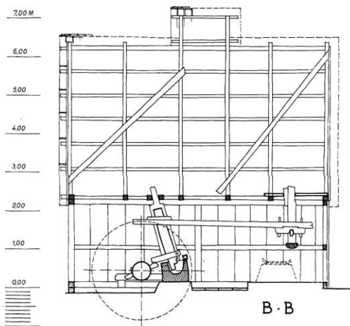
102. ábra. Nyeleskalapácsos kallómalom felmérési rajza (Románia, Dobra Sugag, 1960. Felmérte: Pongrácz Pál)
