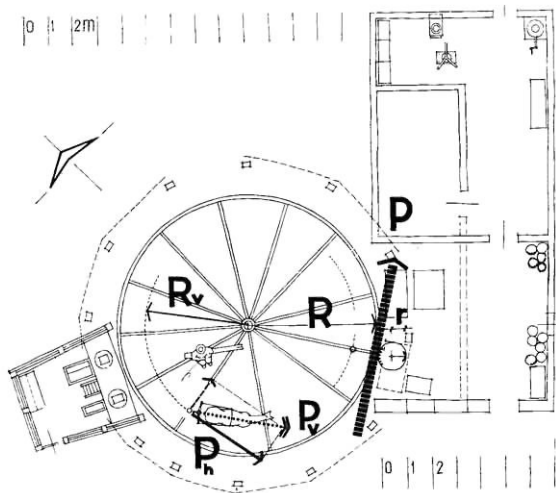
18. ábra Járgányos szárazmalom energiahasznosítása
