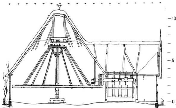
36. ábra Járókerék alatt vontatott gabonaőrő — kendertörő szárazmalom felmérési rajza (Németország, Kniendorf, épült 1797-ben. A. Jespersen: Report on Watermills)
