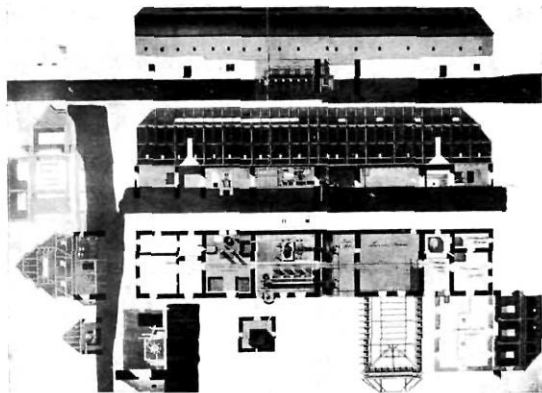
7. ábra Papírmalom tervrajza a XIX. század első feléből (Műszaki Múzeum tervrajgyűjteményéből)
