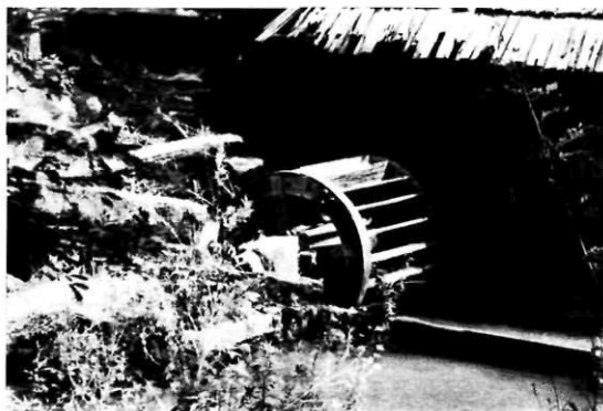
48. ábra. Merülő széles lapátú vízkerék (Románia, Arcani, 1960.)
