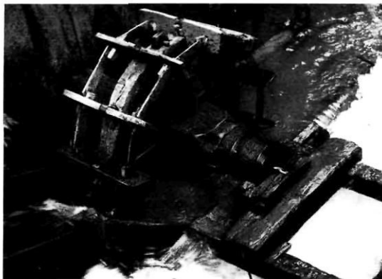
45. ábra Egypereces, keresztküllős, kétoldalt gyámoltott lapátú vízikerek (Románia, Dobra Sugag, 1960.)
