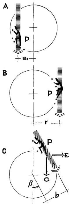
15. ábra. Taposókerekerek A belsőjáratú kerék – a tengelyre ható forgatónyomaték: M = Pa , B külsőjáratú kerék – tengely forgatónyomatéka: M = Pr , C felsőjáratú kerék – a tengelyre ható forgatónyomaték: M = Pb vagy a P komponenseiből ( EG ) adódik
