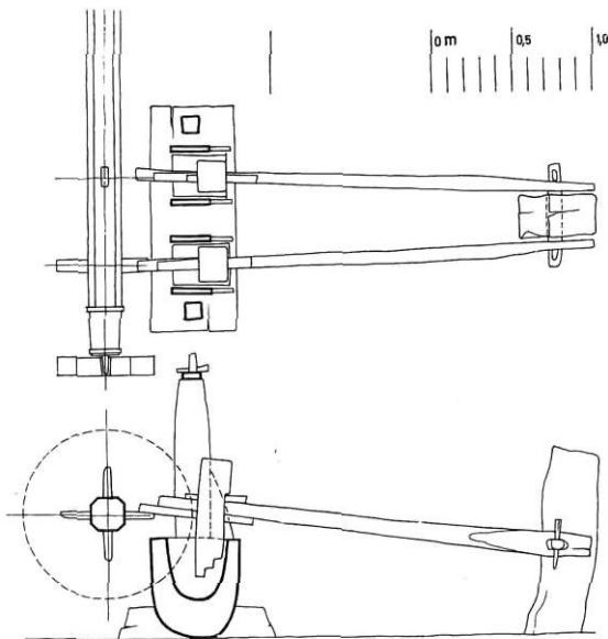
101. ábra Nyeleskalapácsos kallómű (Románia, Jasi Múzeum)
