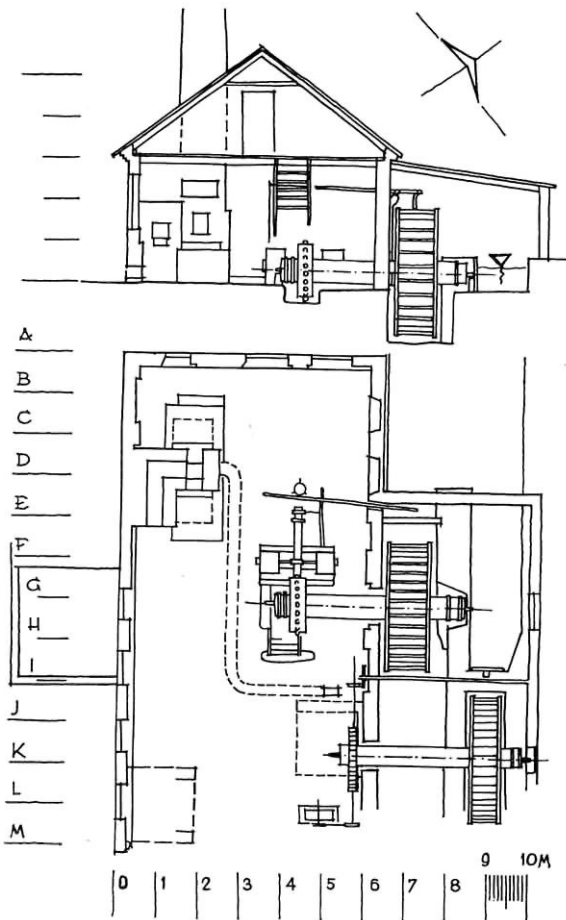
122. ábra. Kalapácsmalom felmérési vázlata (Svédország, Felmérte: Anders Jespersen 1955.)
