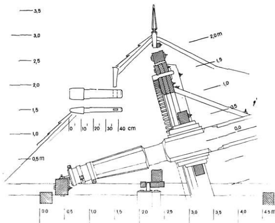
163. ábra. A vitorlatengely és a nagykerék felmérési részletrajza (Szentés — Nagytőke, Csongrád m. Felmérte: Pongrácz Pál 1954.)
