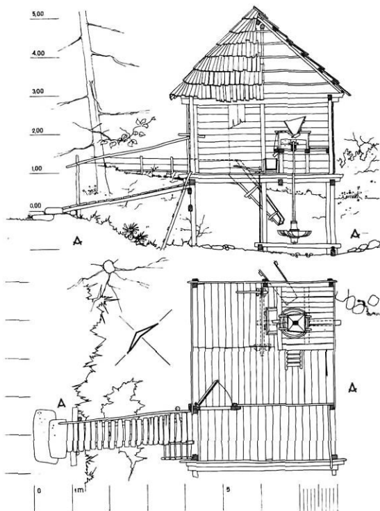
66. ábra Egytengelyes malom felmérési rajza (Románia, Arcani, 1960. Felmérte: Pongrácz Pál)
