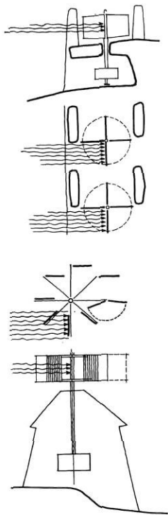
136. ábra Vízszintes síkban forgó vitorlákkal működő malmok egyiptomi partimalom vázlata, és nyíló-csukódó vitorlázatú szélmalom (Verancius, 1595.)
