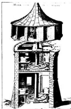
137. ábra Vízszintes síkban forgó vitorladob hajtású malmok (jobb oldal: Verancius, 1595. — bal oldal: Besson, 1578.)
