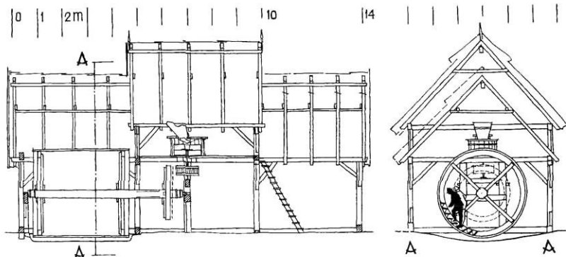
21. ábra. Taposómalom rekonstrukciós rajza
