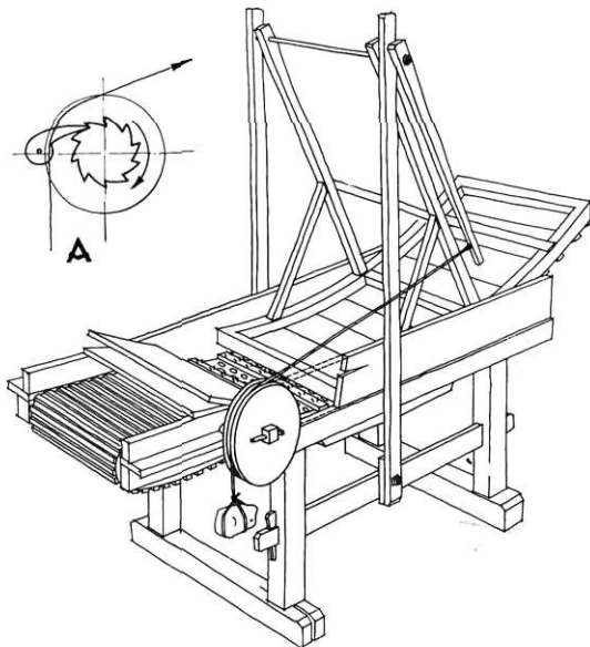
90. ábra. Kézi kártológép
