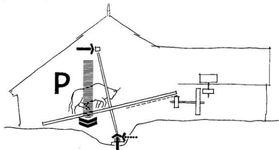
19. ábra. Tiprómalom energiahasznosítása. A függőleges P_t erőből a korong síkjában ható P_h erő P_v komponense képez forgatónyomatékokat a tengelyre
