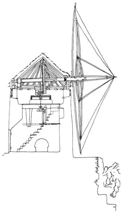
138. ábra. Vászonvitorlás szélmalom metszete és vitorlázata (Görögország; A. Jespersen: Report on Watermills V. 3.)
