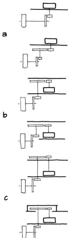
72. ábra. Energiatovábbító berendezések rendszere vízerővel működő gabonaőrőlmalmoknál a alul hajtó, b középen hajtó, c felül hajtó
