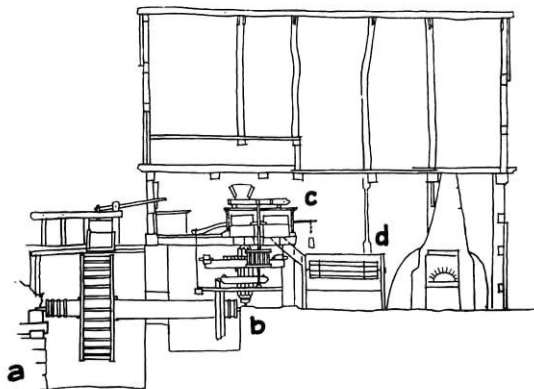
71. ábra. Vízimalom szerkezeti rendszere a vízikerek, b áttételek, c őrlőmű, d szita
