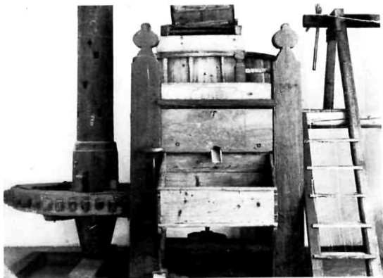
171. ábra Egykőves szélmalom hajtószerkezete és kőpadja (Kiskunfélegyháza, Kiskun Múzeum)
