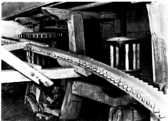
30. ábra. Járószín malomház felőli része a nagykerékkel és az orsókkal (Szarvas, Tonka-féle szárazmalom)
