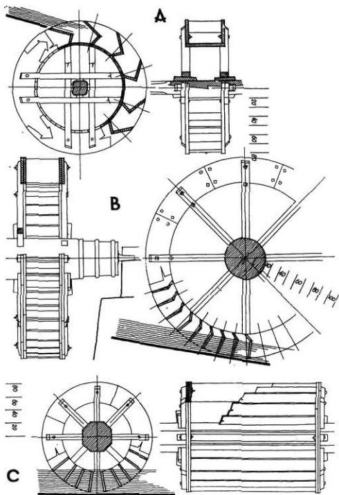
57. ábra Vízikerekek felmérési rajza A járomküllös szekrényes felül csapott vízikerek, B kétpereces, hajlított lapátú vízikerek, C merülő, széles lapátú vízikerek
