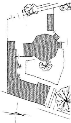
26. ábra. A szarvasi Tonka-féle szárazmalom beépítési vázlata
