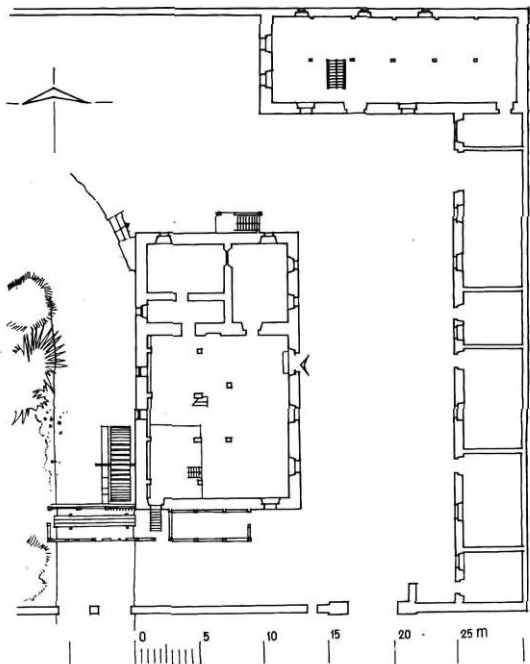
76. ábra Nepomucenus-malom felmérési rajza (Országos Műemléki Felügyelőség tervtára)
