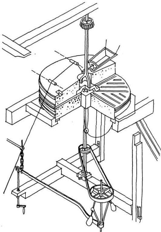
172. ábra Szélmalom őrlőszerkezeté- hez kapcsolódó forgás- szabályozó (Anglia, Rex Wailles The English Windmill)
